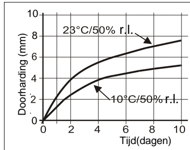
Schema 1: Uithardingsnelheid Sikaflex®-521 UV
